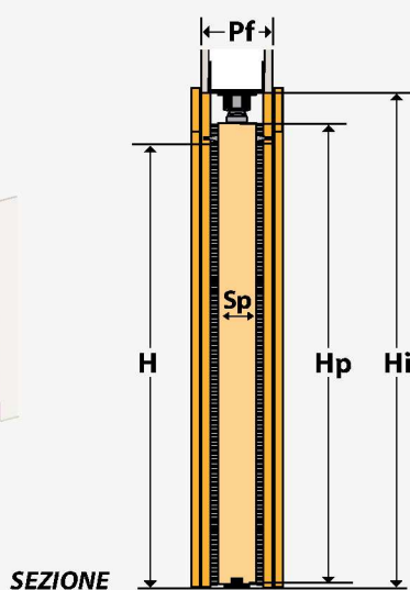
SEZIONE
